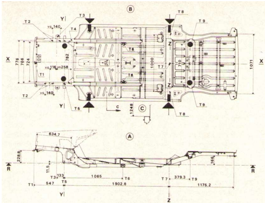
Abb. 3: Rahmenbaugruppe [Werkfoto]
